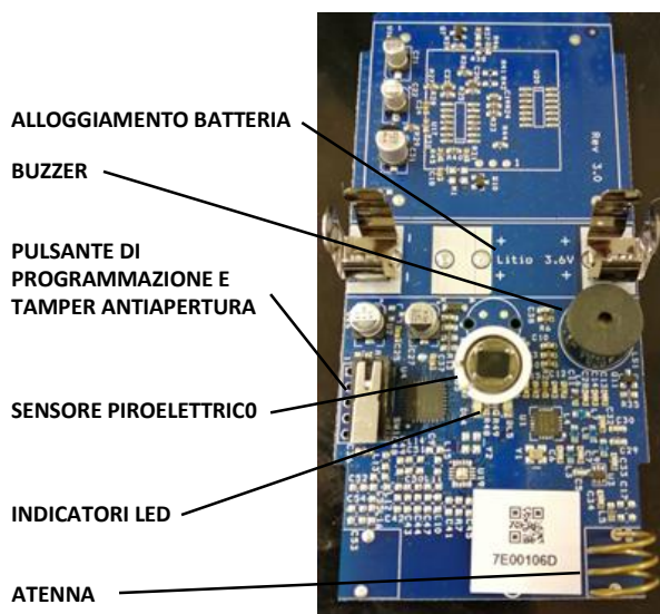
FIG. 2: Scheda Sensore WIR
